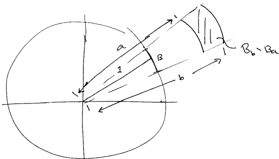
Fig. 22.7. The region B_b \setminus B_a .
