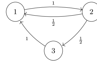
Fig. 21.6. A simple 3 state jump diagram.
